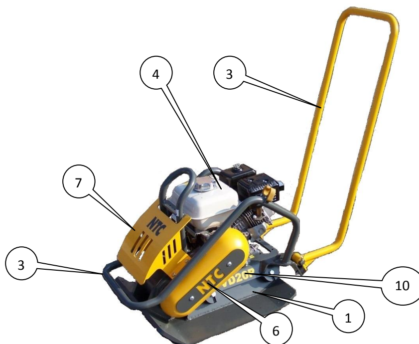
Obr. Základní popis stroje – varianta bez kropíčního zařízení
