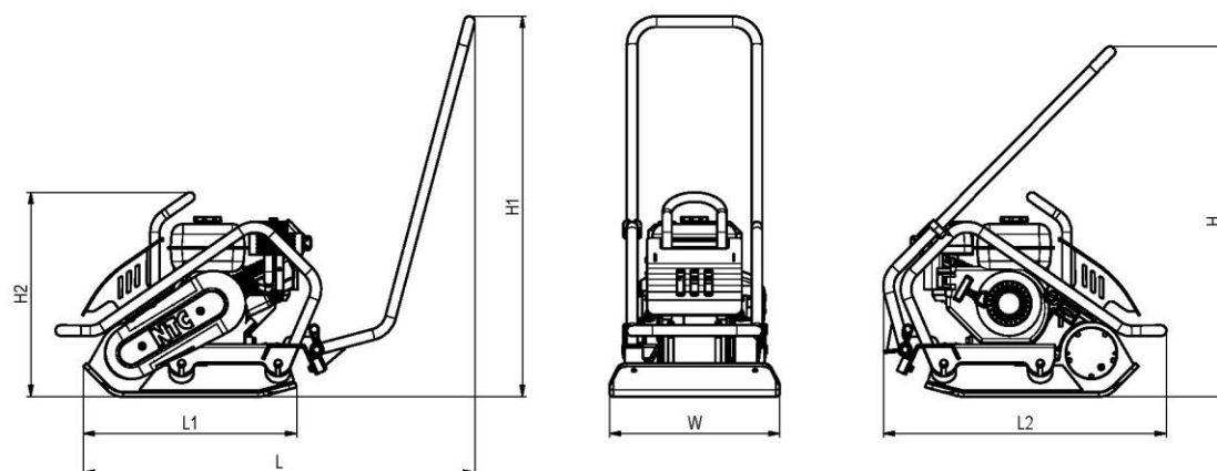
Obr. Základní popis stroje – varianta bez kropíčního zařízení
